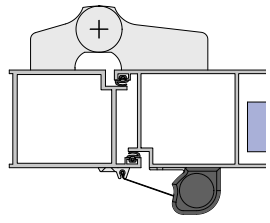
FP800 Dimensions
